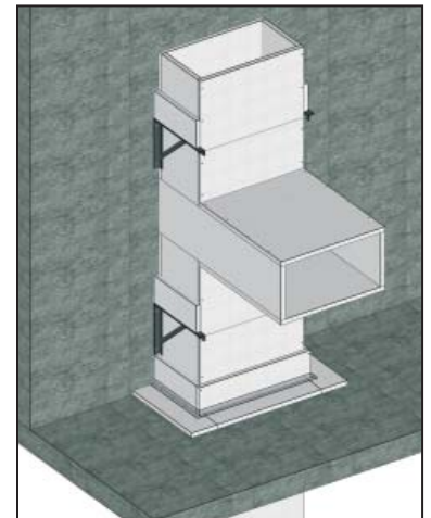
7. Anclaje vertical y empalme horizontal.
